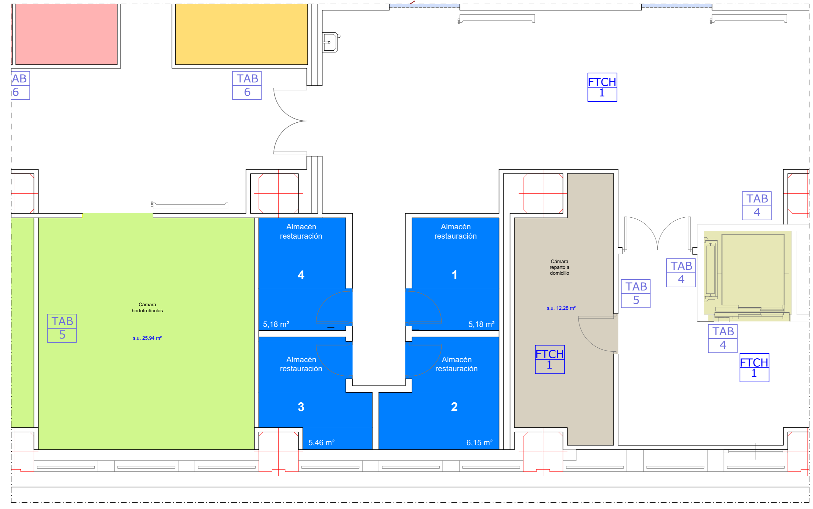
DETALLE ZONA ALMACENES DE RESTAURACIÓN Escala 1:50
